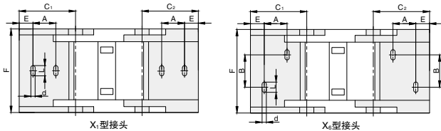
X 1 型接头
