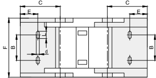
X 2 型接头
