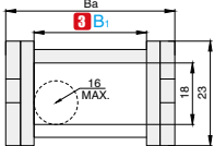
接头安装尺寸图
