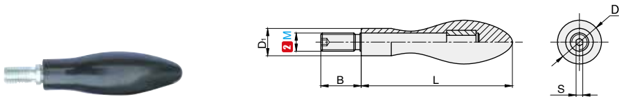
PLEA 曲面转动手柄-A系列
